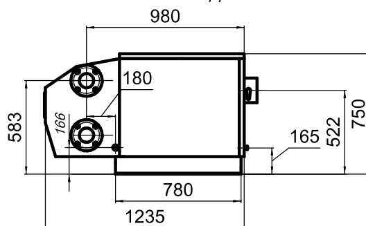
Вид А
