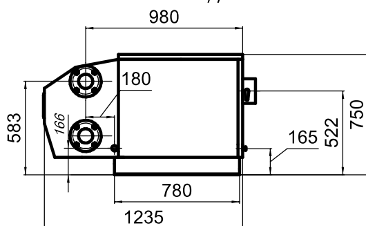
Вид А
